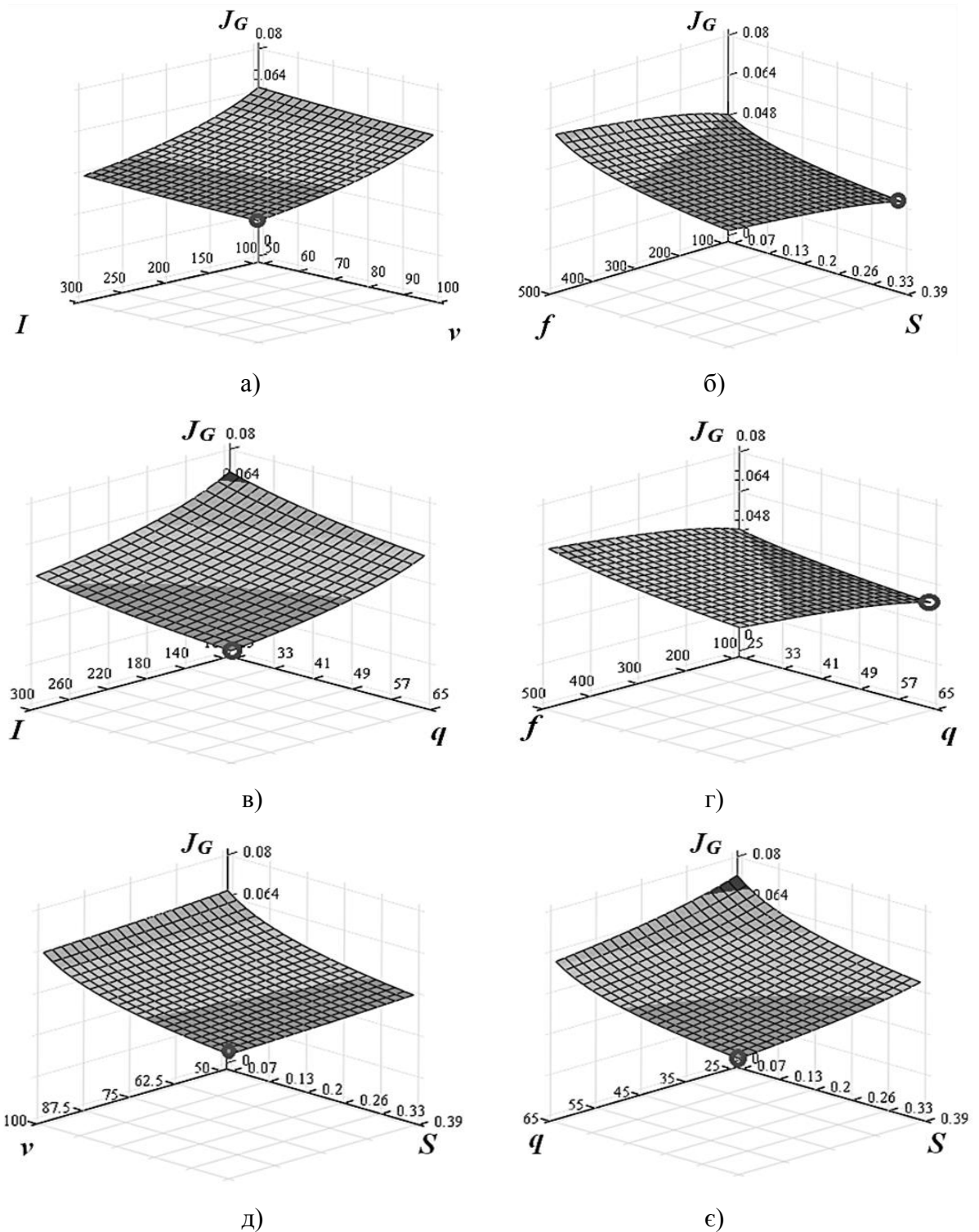
Рис. 2. Координата точки (виділена колом), при якій функція J_G приймає min : а – J_G(I, v) ; б – J_G(f, S) ; в – J_G(I, q) ; г – J_G(f, q) ; д – J_G(v, S) ; е – J_G(q, S)
