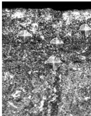
Рис. 1. Мікроструктура зразка зі сталі 40ХН (x125), обробленого точінням з ЕІН
